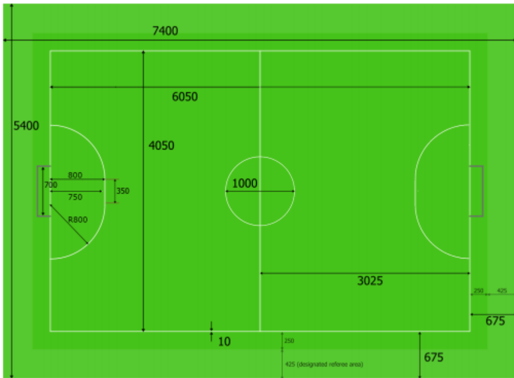
图 4-1 小型机器人足球赛比赛场地尺寸图
